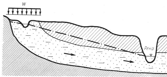
Рис. 3. Схема фильтрации в условиях напорно-безнапорного потока: W — величина инфильтрации; пунктирная линия — пьезометрическая кривая; стрелкой показано направление движения потока
